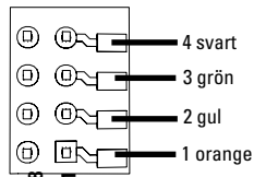
Ovansidans lödpunkter
